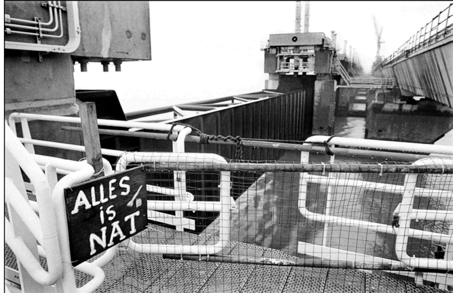
De stormvloedkering in de Oosterschelde nadert haar voltooiën. Het is een van de huzarenstukjes van het deltaplan tegen overstroming van zuidwest Nederland.
